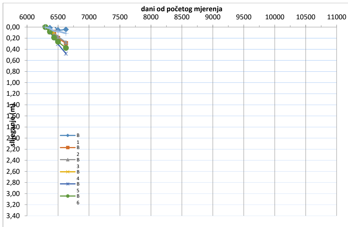
Slika 8. Prikaz konsolidacije repera broj B1, B2, B3, B4, B5, B6, B7 (profil 14). Horizontalna os prikazuje vrijeme u danima, a vertikalna os prikazuje slijeganje u metrima. Vrijeme je prikazano u linearnom mjerilu. Početni datum mjerenja slijeganja je 21.02.2024.
