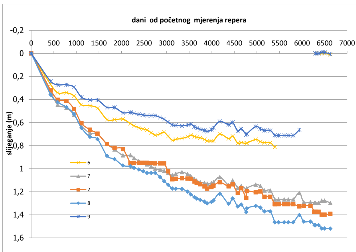
Slika 1. Prikaz konsolidacije repera broj 2, 6, 7, 8, 9 (profil 2). Horizontalna os prikazuje vrijeme u danima a vertikalna os prikazuje slijezanje u metrima. Vrijeme je prikazano u linearnom mjerilu. Početni datum mjerenja slijezanja je 24.11.2006.
