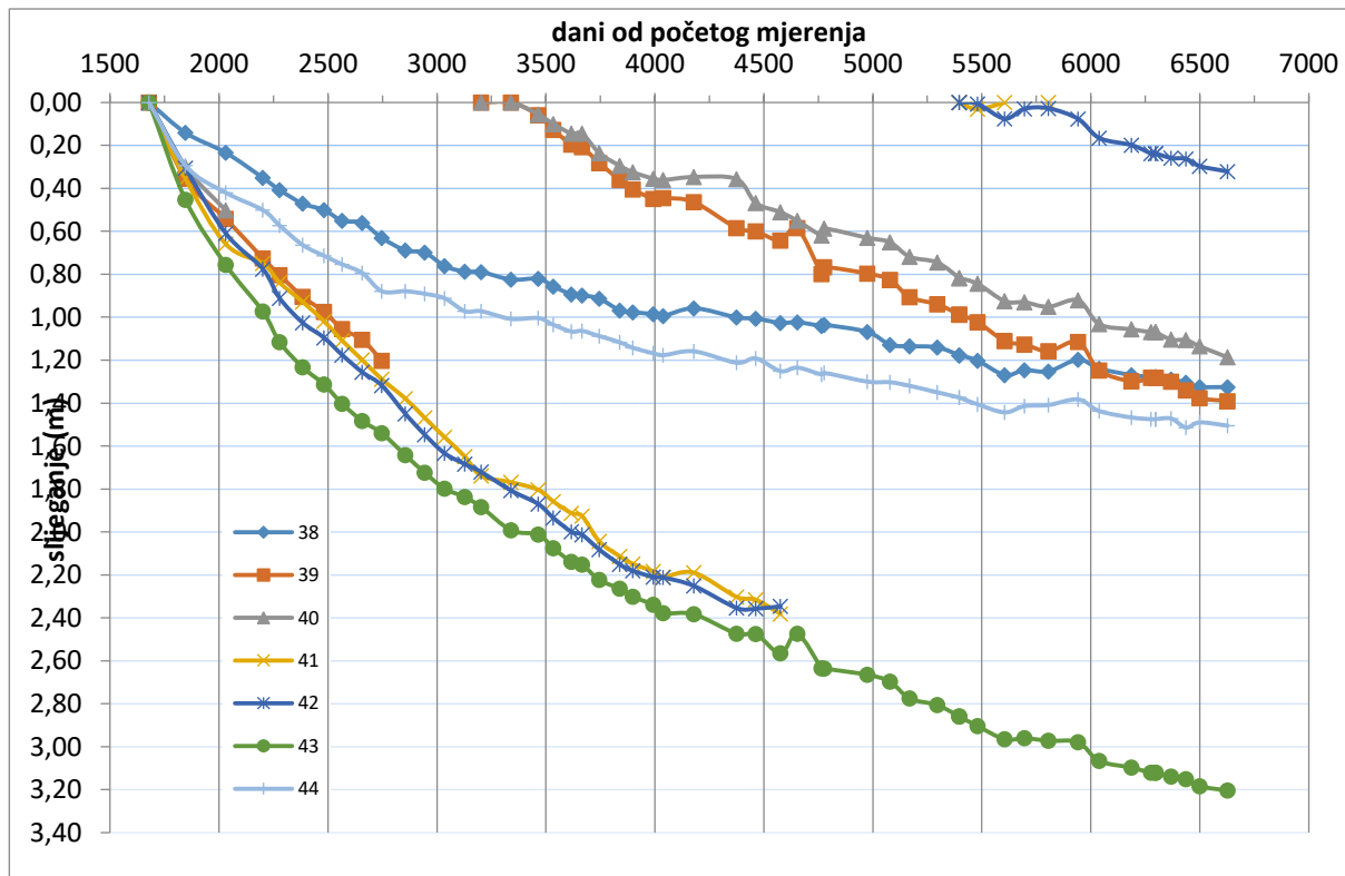
Slika 7. Prikaz konsolidacije repera broj 38, 39, 40, 41, 42, 43, 44 (profil 12). Horizontalna os prikazuje vrijeme u danima, a vertikalna os prikazuje slijezanje u metrima. Vrijeme je prikazano u linearnom mjerilu. Početni datum mjerenja slijezanja je 30.06.2011. Početni datum mjerenja slijezanja repera br. 42 je 03.09.2021.
