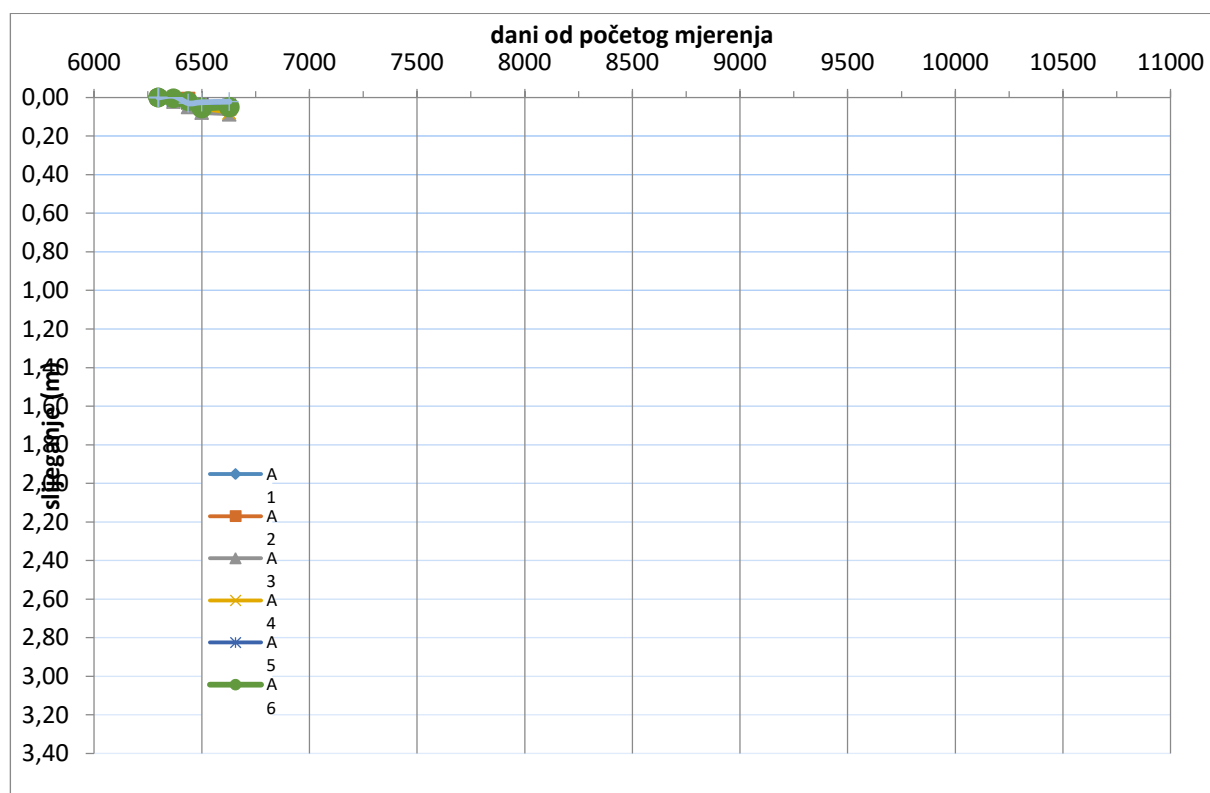
Slika 6. Prikaz konsolidacije repera A1, A2, A3, A4, A5, A6 (profil 11). Horizontalna os prikazuje vrijeme u danima a vertikalna os prikazuje slijeganje u metrima. Vrijeme je prikazano u linearnom mjerilu.
